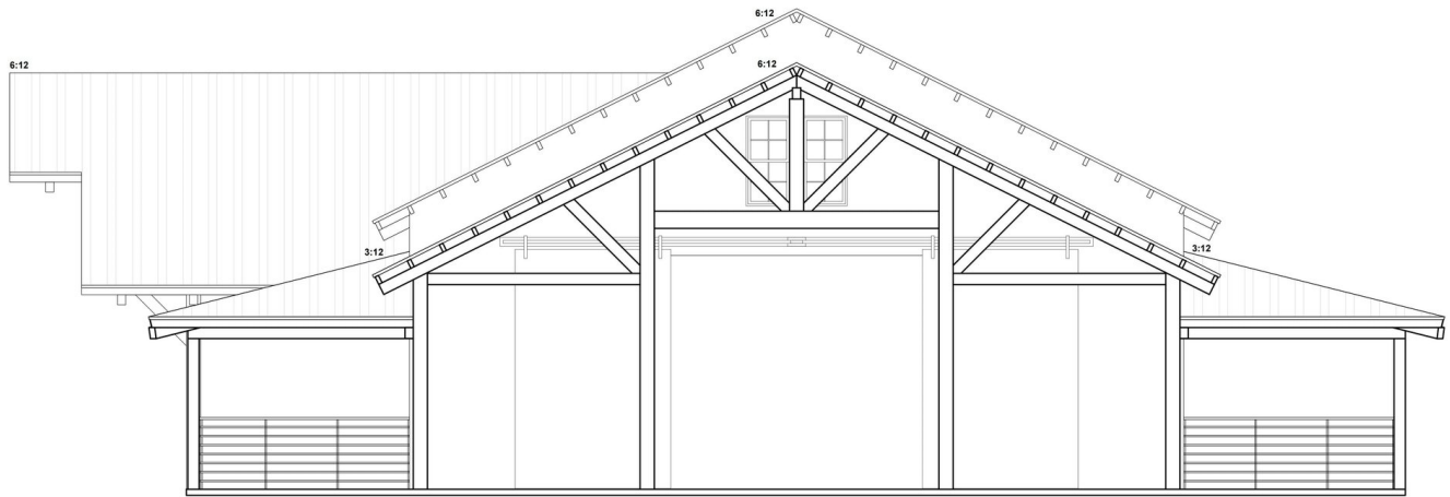
RIGHT ELEVATION
