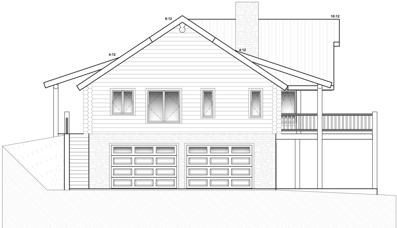
RIGHT ELEVATION
