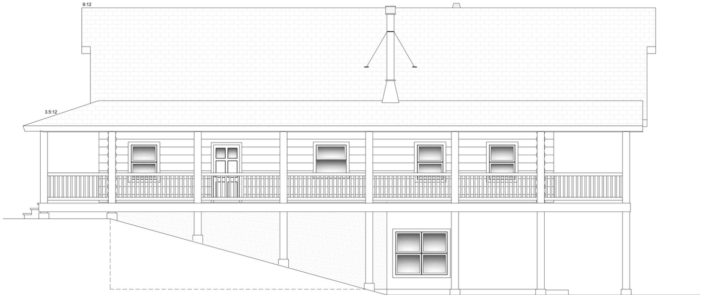
RIGHT ELEVATION
