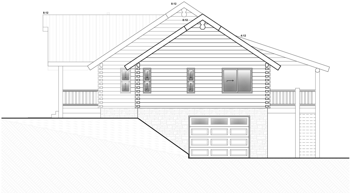
RIGHT ELEVATION
