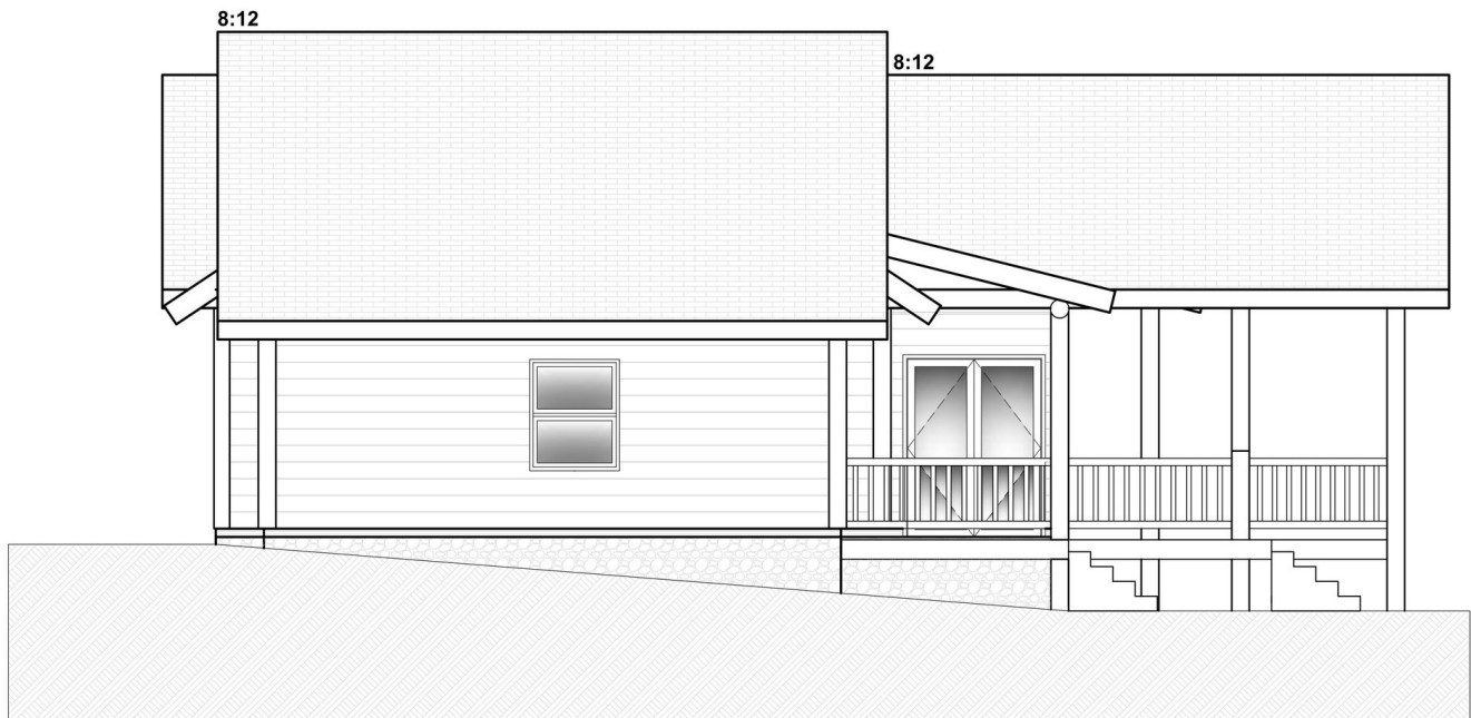
RIGHT ELEVATION
