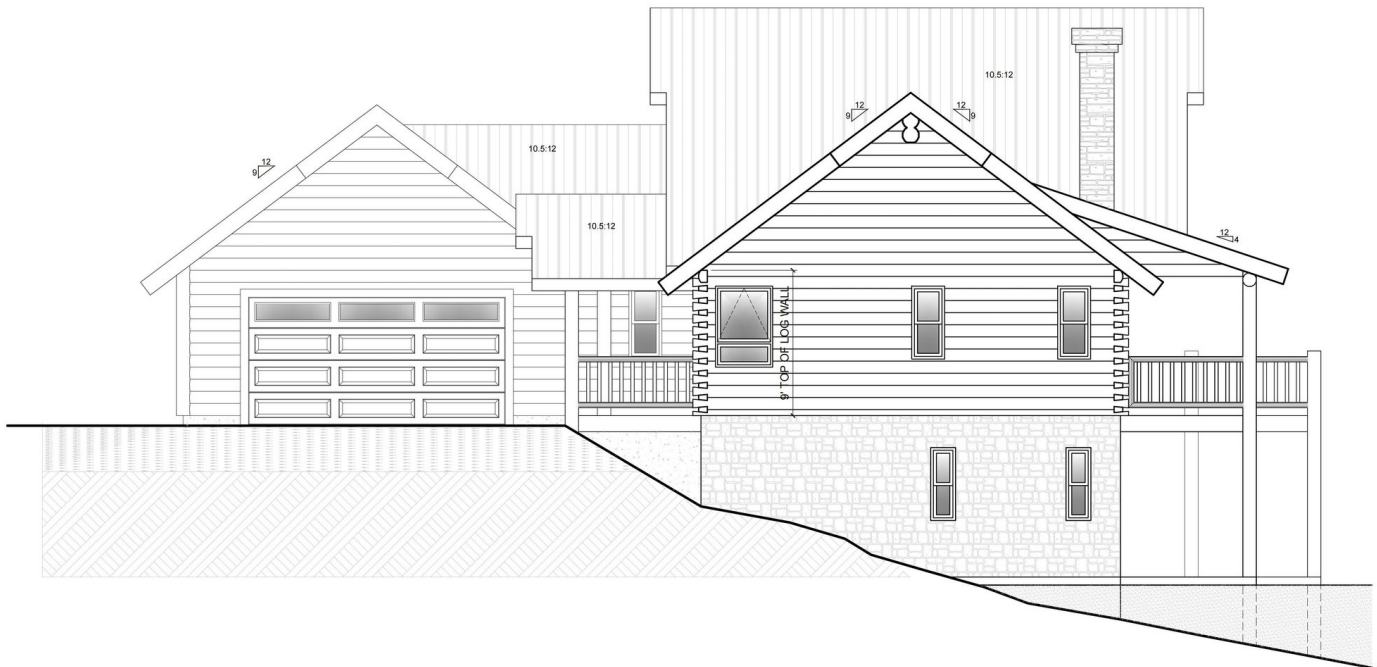
RIGHT ELEVATION
