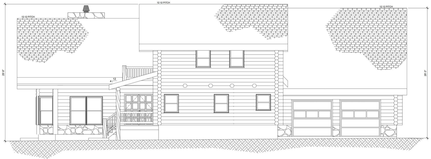
RIGHT ELEVATION
