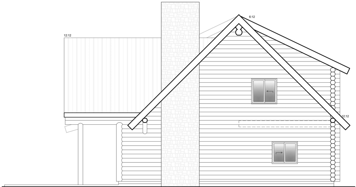
RIGHT ELEVATION
