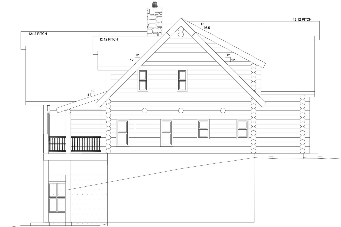
RIGHT ELEVATION
