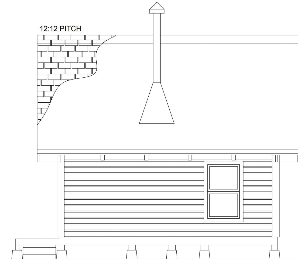
RIGHT ELEVATION
